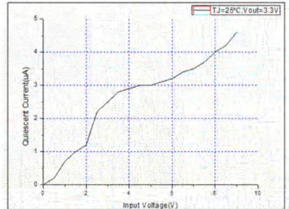
图2 静态功耗和输入电压关系
